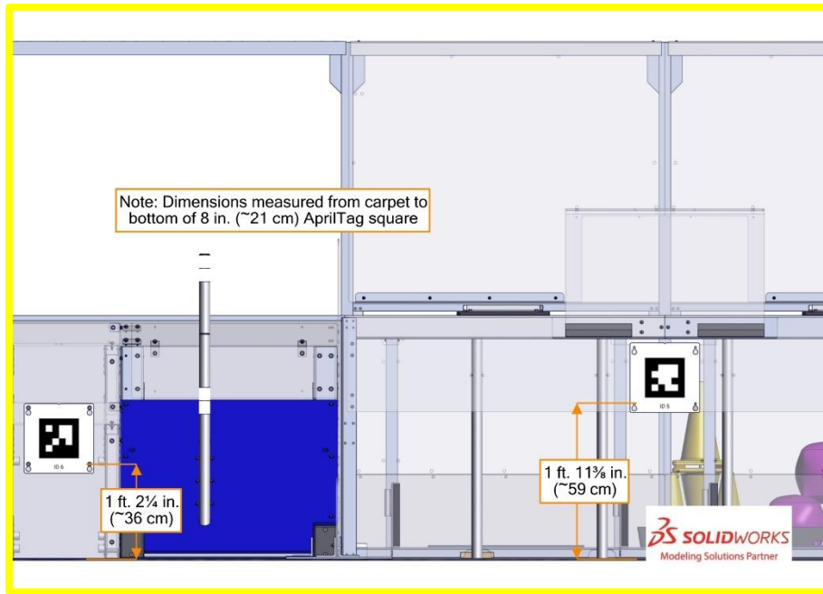
Şekil 5-33 AprilTag konumlandırma boyutları
